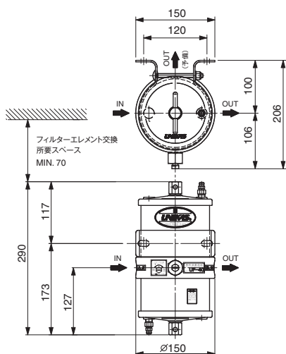
外形寸法図
